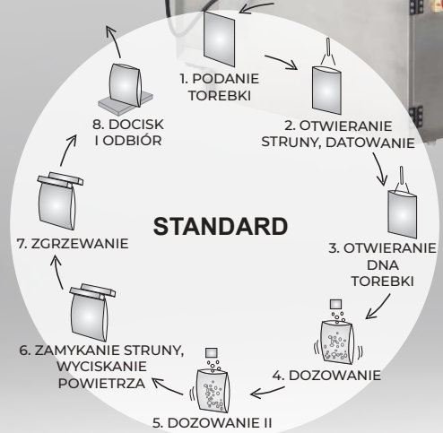
Automat pakujący COFFPACK DOYPACK K 8-45
