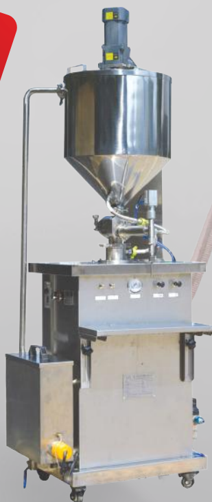
Dozownik wolnostojący płynów gęstych DWPG/S HOT (system podgrzewania HOT)
