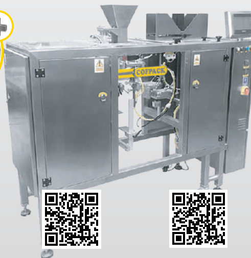
Automat pakujący COFPACK MULTI 160/300 U/ SC
